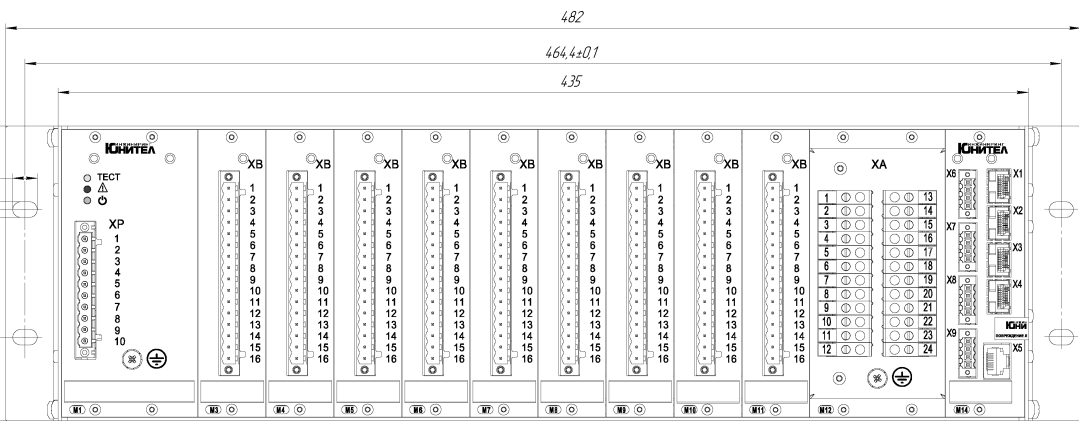
Рисунок Г.1 – Габариты и установочные размеры устройства в исполнении ЮНИТ-М319-Д3Т2 (I архитектура)
